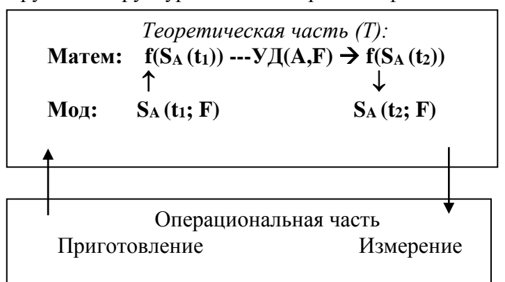
Сх. 3. Структура теоретического описания 1) оснований раздела физики (при A=П ИО) и 2) физического процесса (при A=В ИО). f(S_A(t_1)) означает математический образ S_A(t_1)
